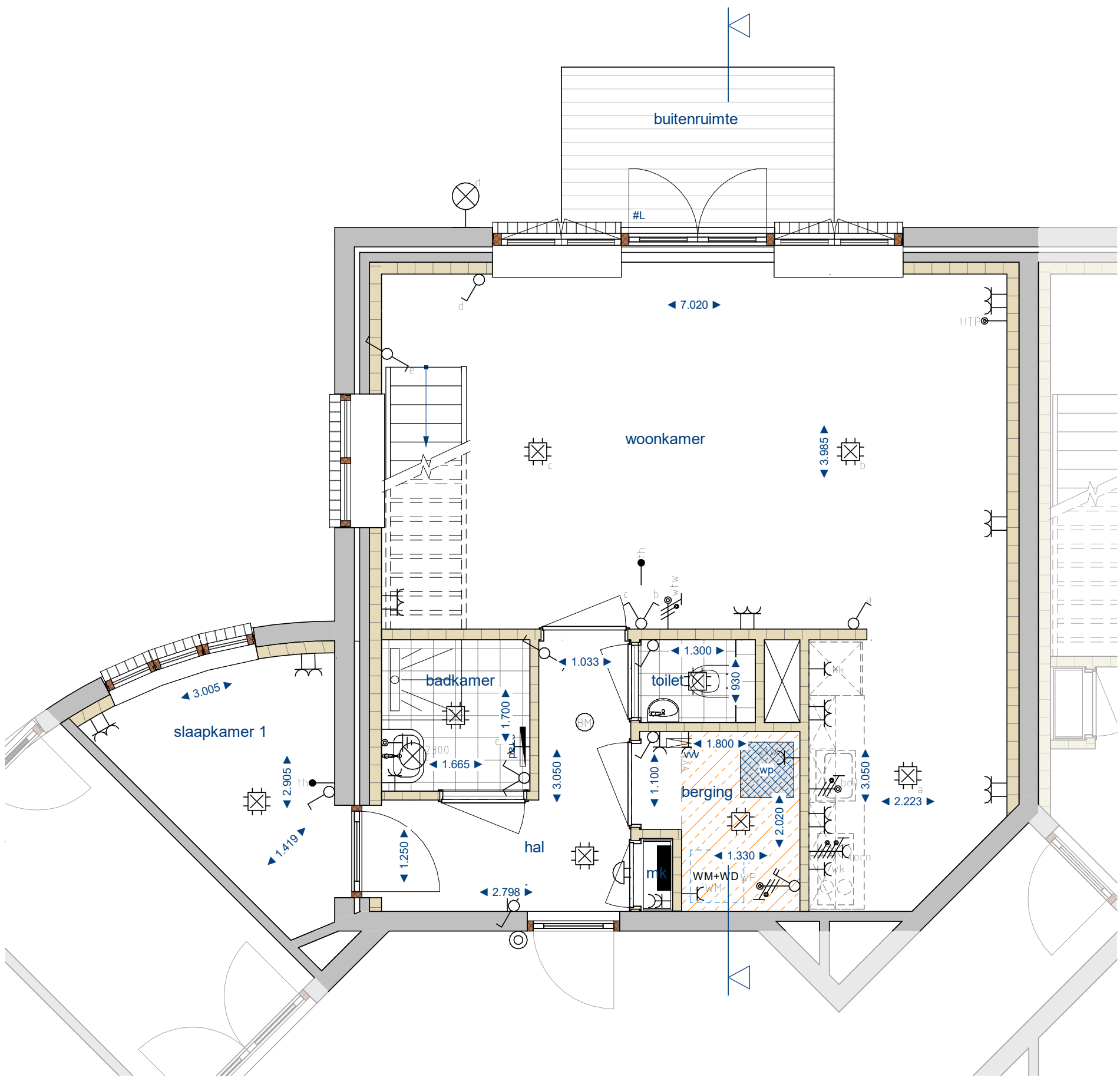
begane grond
