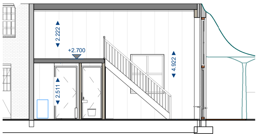
doorsnede
